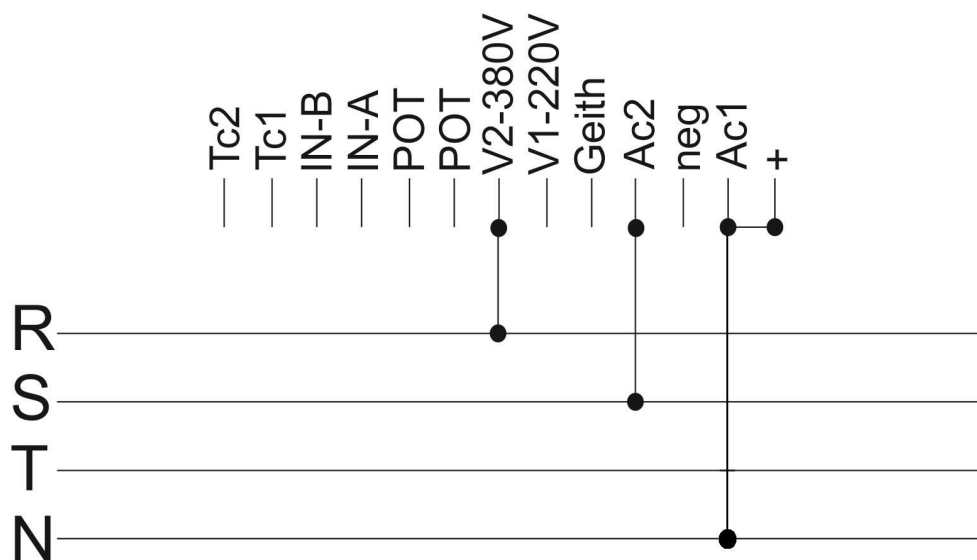
Ligação em 380V - FFN = Fase - Fase - Neutro
