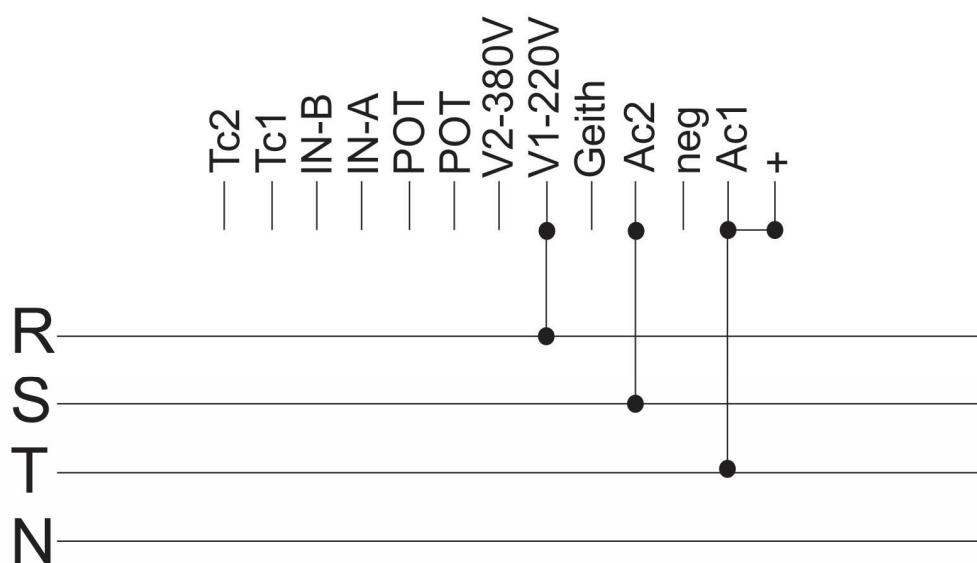
Ligação em 220V - 3 fases
